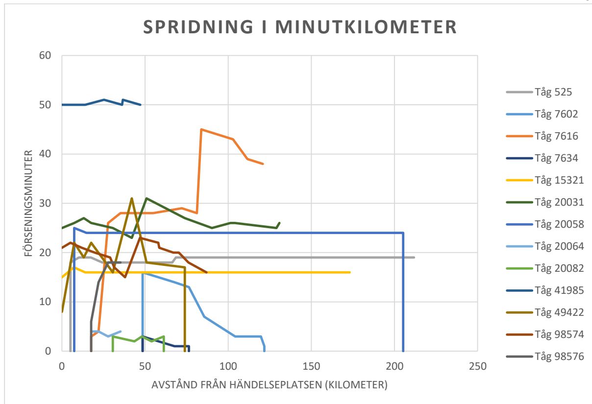
Figur 13 Störningspridning i kilometer avstånd från händelseplatsen
