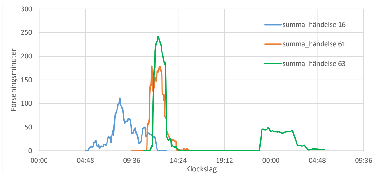
Figur 16: Summa av total förseningsminuter för varje händelse
