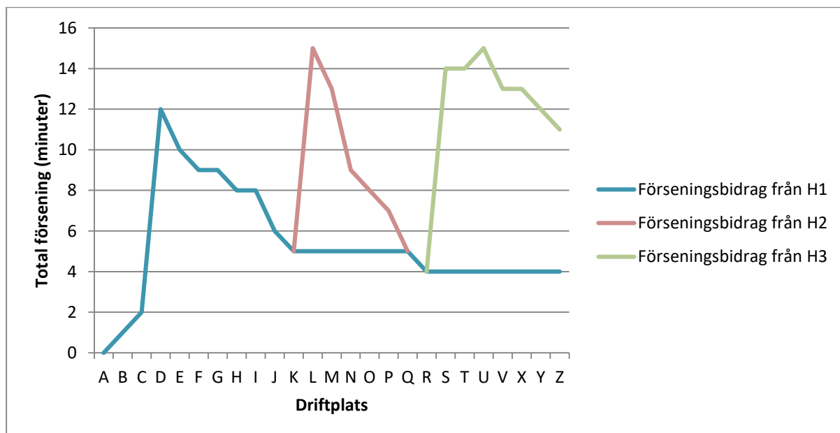
Figur 9: Fördelning av försening och återhämtning till olika händelser. Återhämtning och oregistrerad merförsening kopplas alltid till den senaste registrerade händelsen/merförseningen som ger ett förseningsbidrag.
