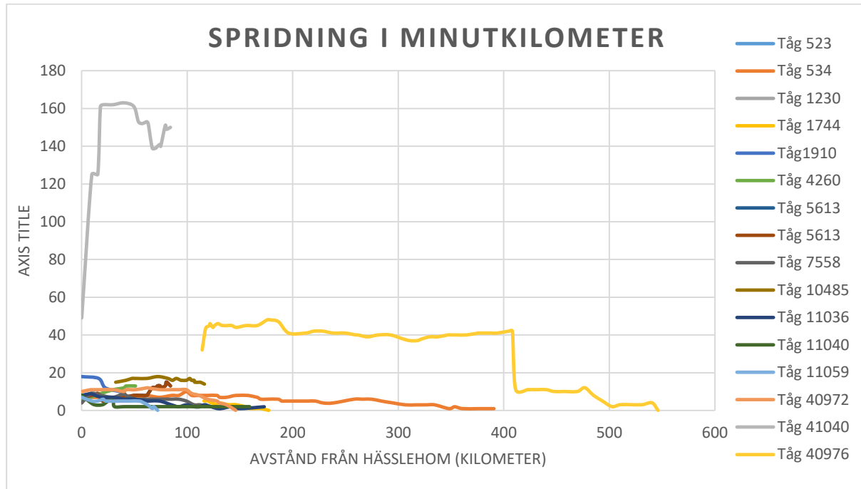
Figur 25 Alla tågs förseningar som associerats till händelsen i Markaryd-Hässlehom. x-axeln visar spridnings avstånd från Hässlehom.
