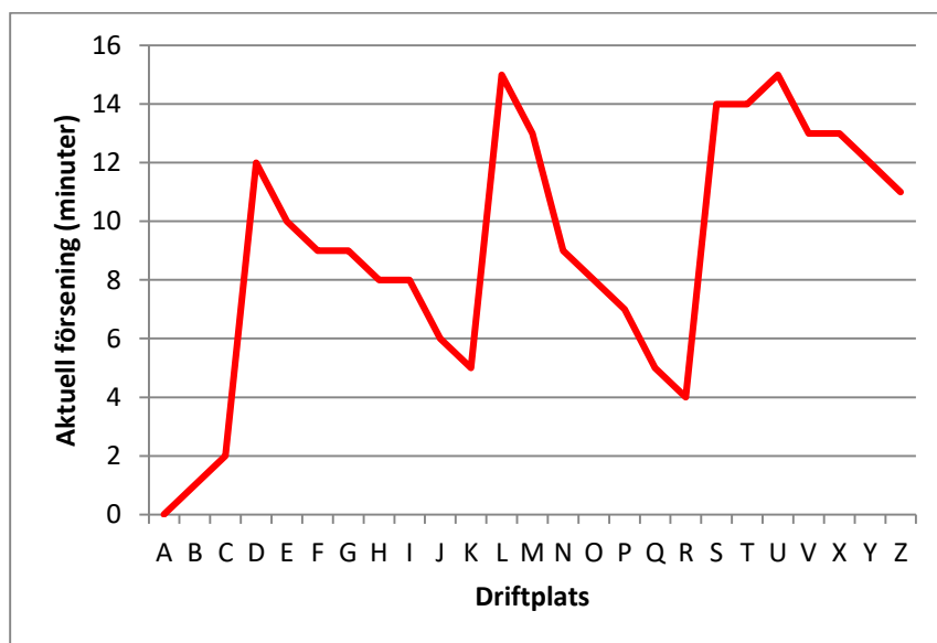
Figur 7: Diagram illustrerande försening för exempeltåget 4711 vid en fiktiv resa från station A till Z. Vid driftplatserna D, L och S inträffar oberoende händelser (kallade H1, H2 och H3) som ger upphov till merförseningar på 10 minuter vardera. Dessutom finns mindre ("oregistrerade") merförseningar.
