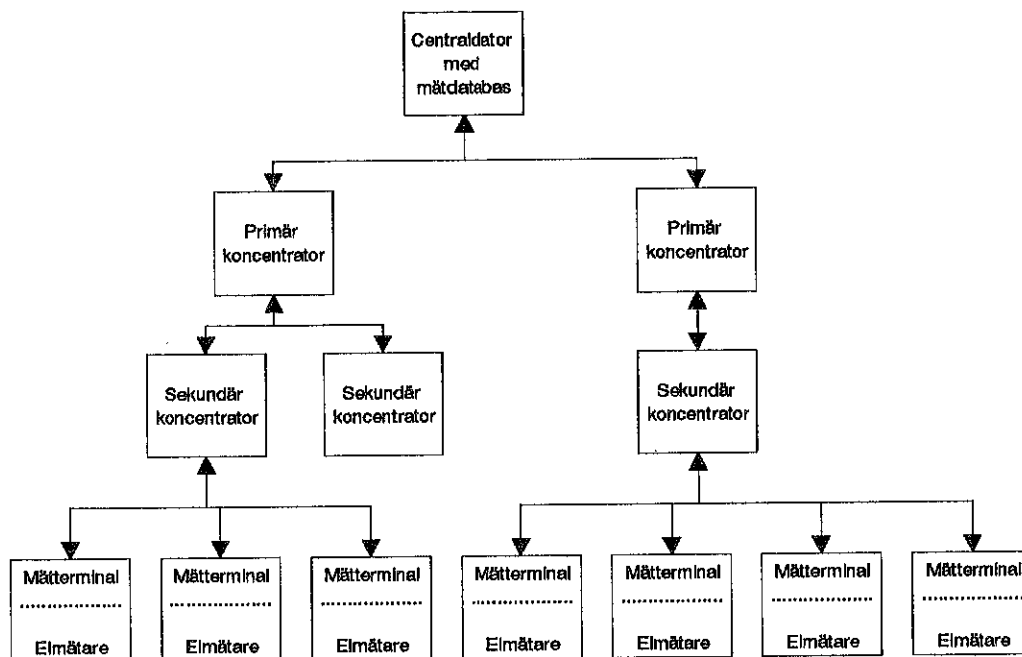
Figur 3. Princip för RCM-systemets logiska uppbyggnad.
