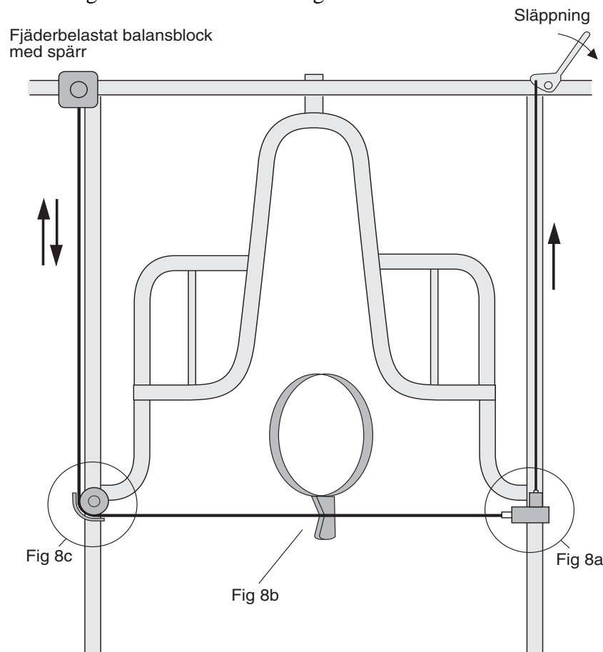
Figur 2. En lina löper mellan båsfrontens sidorör, 30 – 60 cm över båsfallens nivå. Linan spänns med en vajerkassett.
